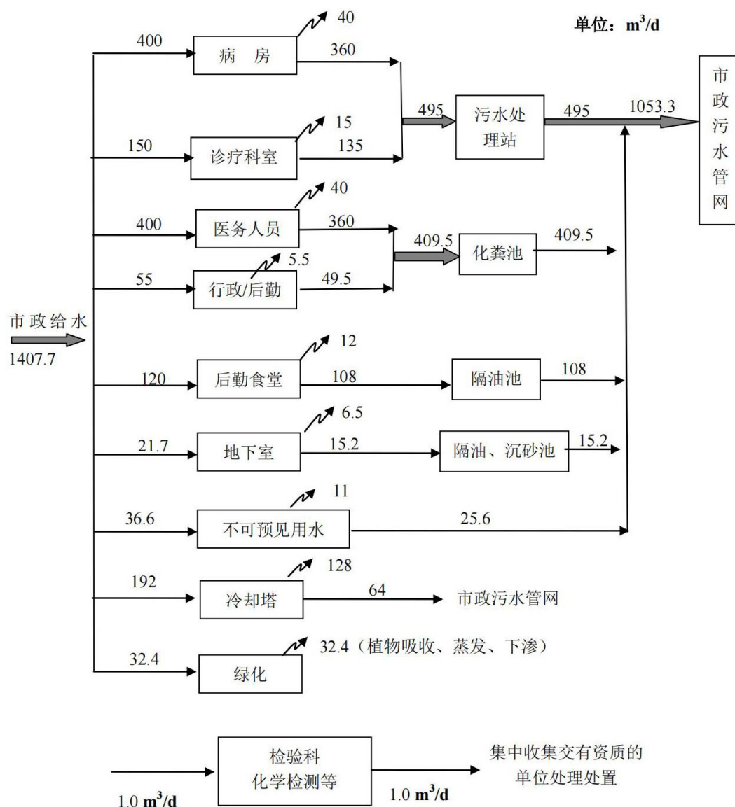
图 3.3-1 环评阶段项目用水平衡图（单位: m 3 /d）
